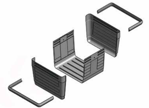
El cuerpo del contenedor RST está compuesto solo por tres piezas principales: las dos laterales y una banda única continua interna.
